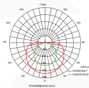
· 配光曲线图
